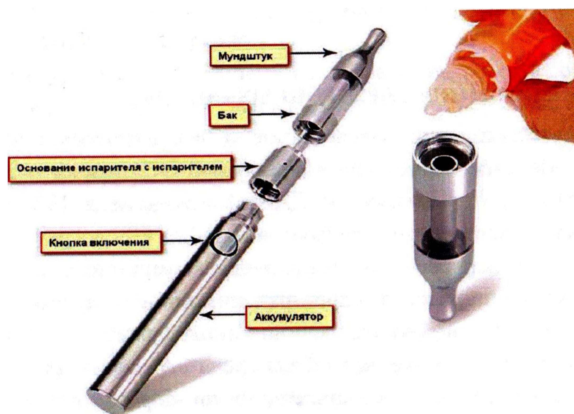
Рис. 3. Устройство электронной сигареты
